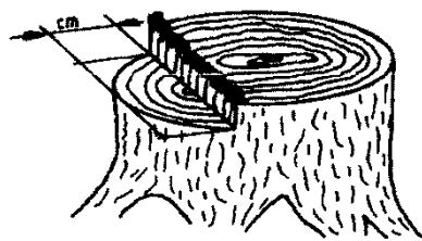
Abb. 3 Fallkerbtiefe 7 cm – 12 cm
